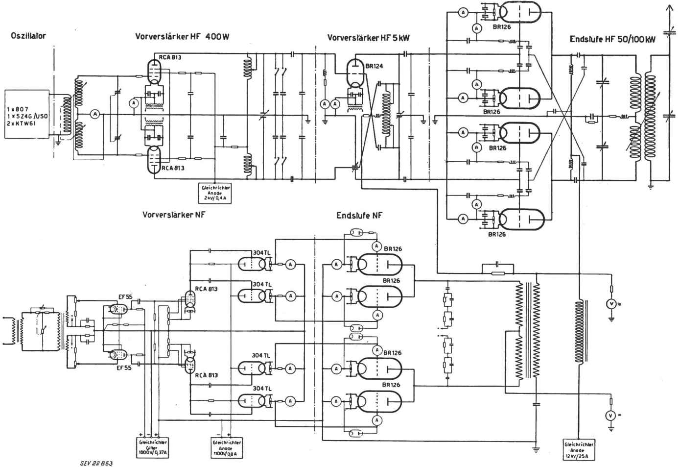
Fig. 1 Prinzipschema des Senders Monte Ceneri
