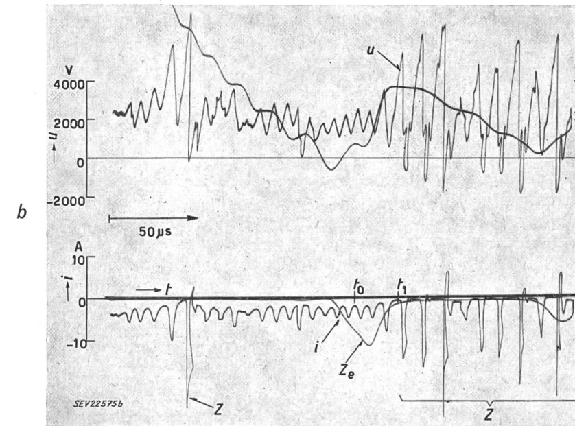
Fig. 5 Verlauf des Lichtbogenstromes und der Lichtbogen-Spannung beim Abschalten eines induktiven Stromes von 41 A bei 24 kV und 50 Hz mit einem Druckluft-schnellschalter
