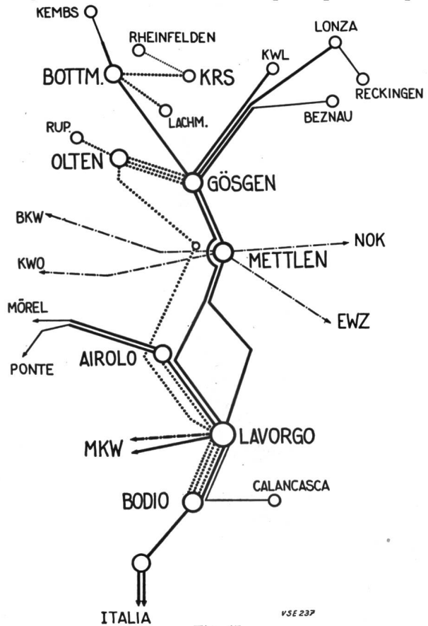
Fig. 17 Réseau téléphonique appartenant en propre à l'ATEL appartenant à l'ATEL appartenant à des tiers — — liaisons en haute fréquence ..... ..... liaisons en basse fréquence - - - - - - - - - - liaisons en haute fréquence } projetées o-o-o-o-o o-o-o-o-o liaisons en basse fréquence
