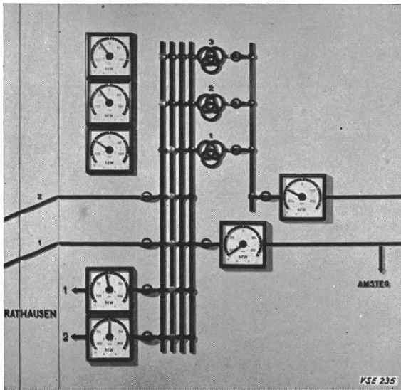
Fig. 15 Partie du schéma du répartiteur de charge de Mettlen
