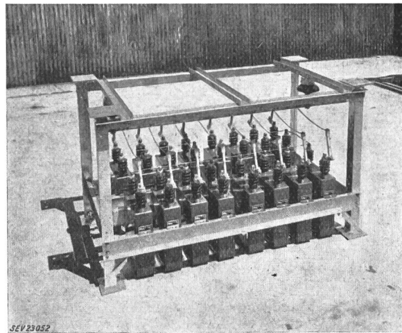
Fig. 2 400-kVar-Block-Einheit mit 16 Kondensatoren (Näheres siehe in Abschnitt 5)
