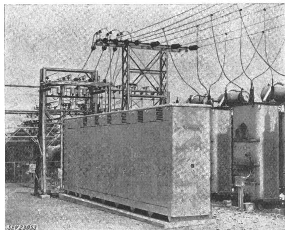
Fig. 3 Verschaltete Kondensatorbatterie von 5400 kVar, 7,2/12,5 kV (Näheres siehe in Abschnitt 5)
