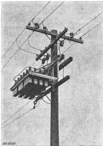
Fig. 1 300-kVar-Kondensatorbatterie auf einem Leitungsmast einer 2,4/4,16-kV-Leitung (Näheres siehe in Abschnitt 5)
