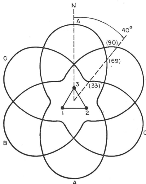
Fig. 1 Navaglobe-Ausbreitungs-Charakteristik
