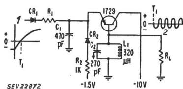
Fig. 1 Amplituden-Komparator mit abgestimmtem Kreis Resonanzfrequenz 400...500 kHz 1 Eingang; 2 Ausgang
