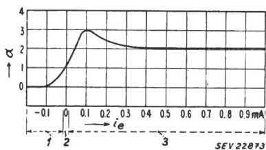
Fig. 2 Verhältnis \alpha von Kollektor- zu Emitterstrom in Funktion des Emitterstromes i_e eines typischen Spitzentransistors 1, 2, 3 Bereiche
