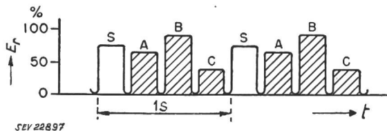
Fig. 2 Navaglobe-Empfangssystem Die gleichgerichteten Signale A, B und C bei einer Peilstellung von 40° S bedeutet das auf leicht verschiedener Frequenz ausgestrahlte Synchronisier-Signal; E_r relative Signalstärke; t Zeit
