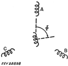
Fig. 3 Schema des Peilrichtungs-Anzeigers
