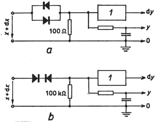
Fig. 10 Schaltungen zur Erzeugung einiger besonderer Funktionen a Funktion in Fig. 9f b Funktion in Fig. 9j 1 Filter Weitere Erklärungen siehe Text
