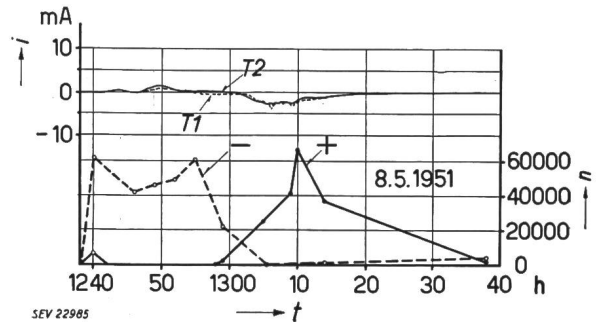
Fig. 10 Verlauf der Ionendichte und des gleichzeitigen Glimmstromes an Turm T1 und T2 1. Beispiel
