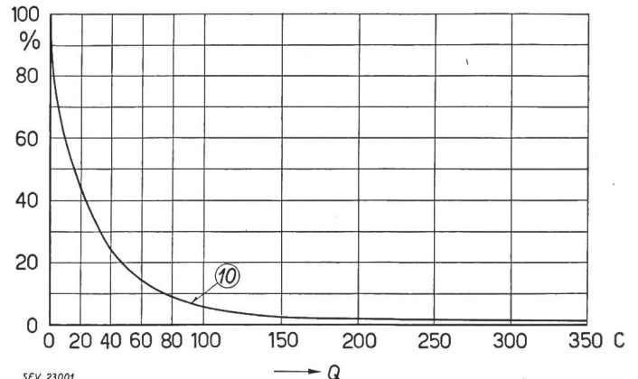
Fig. 26 Häufigkeit der Ladungen von Gesamtblitzen Q Ladung
