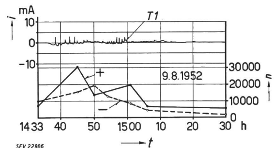
Fig. 11 Verlauf der Ionendichte und des gleichzeitigen Glimmstromes an Turm T1 2. Beispiel
