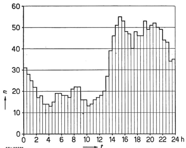
Fig. 3 Tagesgang der Gewittertätigkeit auf dem San Salvatore 1947...1954 n Anzahl Gewitter; t Zeit
