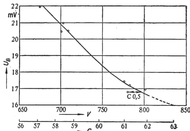
Fig. 3 Eichkurve von acht Lagern V Härte nach Vickers; C Rockwell Härte; U_B Spannung proportional zu B in mV Weitere Bezeichnungen siehe Fig. 1
