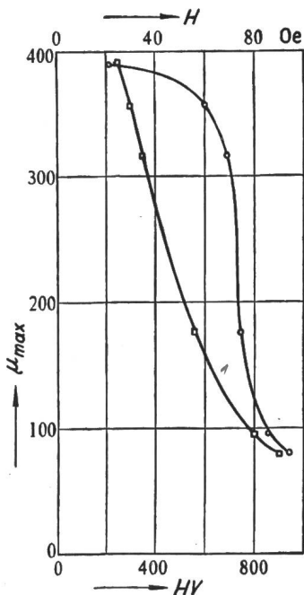
Fig. 2 Zusammenhang zwischen Härte HV, Feldstärke H und maximaler Permeabilität \mu_{max} bei verschiedenen wärmebehandelten Stahlproben HV Härte nach Vickers o \mu_{max} = f(HV) □ \mu_{max} = f(H)
