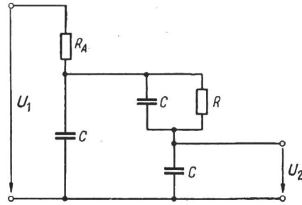
Fig. 2 Der Wiegand-Hansen-Integrator
