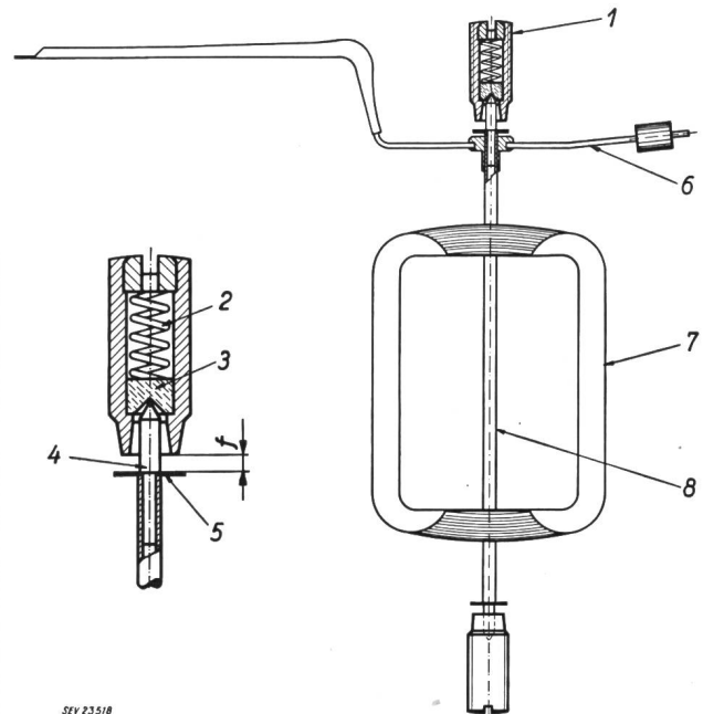
Fig. 8 Spitzenlagerung
