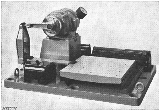
Fig. 2 Vibrationmaschine
