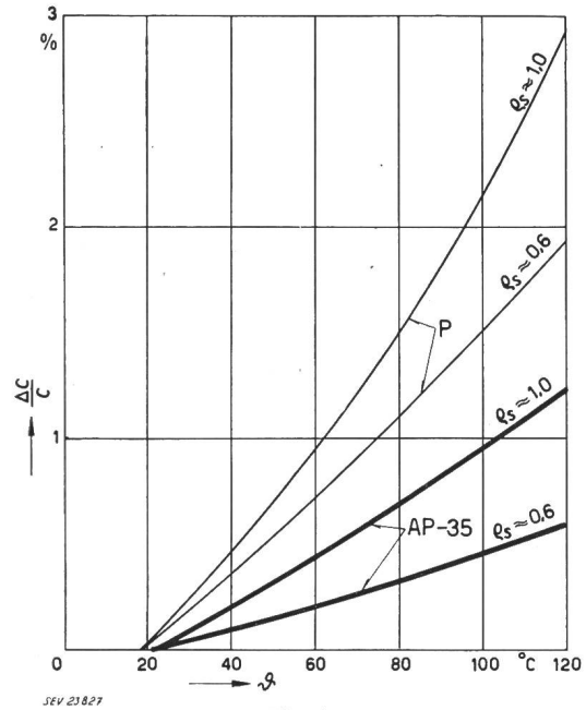
Fig. 17 Relative Kapazitätsänderung \frac{\Delta C}{C} von Zylinder-Kondensatoren in Abhängigkeit von der Temperatur \phi , bei Verwendung von acetyliertem Papier bzw. Kabelpapier als Dielektrikum AP-35 acetyliertes Papier, 35% AcOH P Kabelpapier \rho_s Rohdichte der Blätter in g/cm^3
