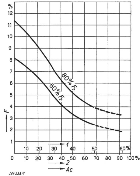
Fig. 7 Reduktion der Feuchtigkeitsaufnahme infolge Acetylierung Feuchtigkeitsgehalt F (in Prozenten des Trockengewichtes) in Abhängigkeit vom Acetylierungsgrad Ac 1 Gehalt an chemisch gebundener Essigsäure (% AcOH) 2 Acetylierungsgrad in Prozenten der total möglichen Acetylierung
