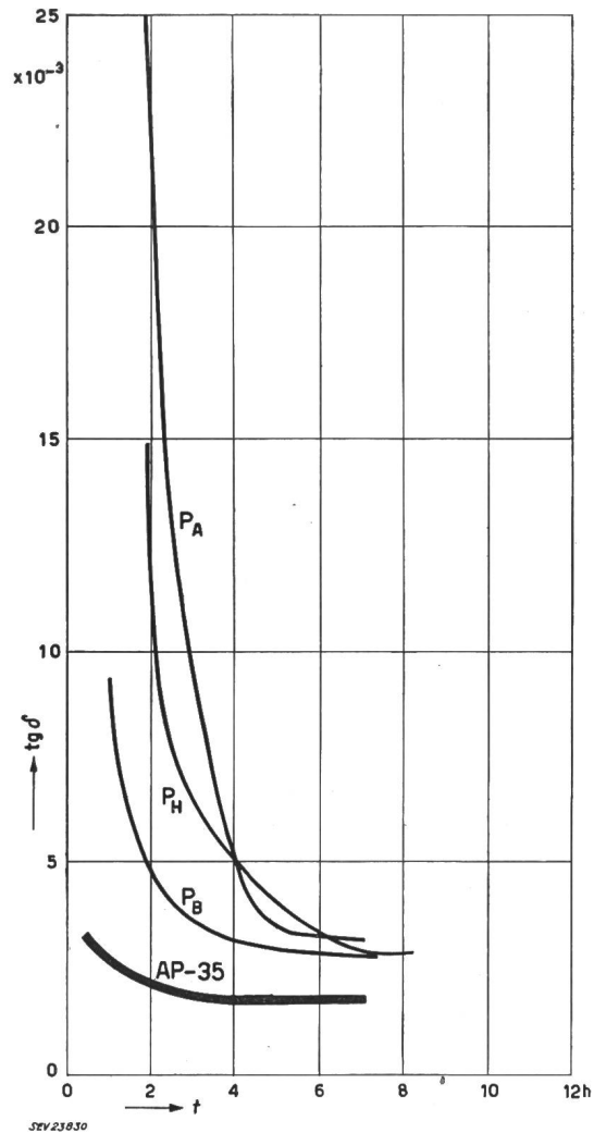
Fig. 20 Verlauf des dielektrischen Verlustfaktors \text{tg } \delta (bei 50 Hz) von verschiedenen Kondensator-Dielelektrika während der Dauer t ihrer Trocknung bei 110^\circ\text{C}
