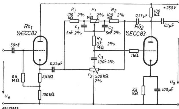
Fig. 1 Entzerrerschaltung
