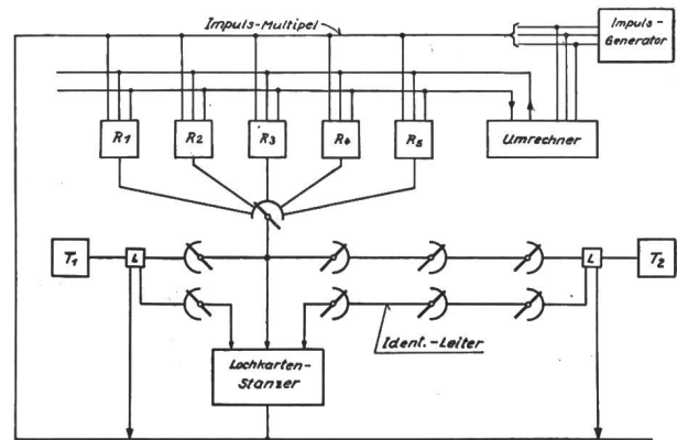
Fig. 8 Anwendungen der Impuls-Identifikation T_1, T_2 Teilnehmer; L Linienstromkreise der Teilnehmer; R_1...R_5 Register
