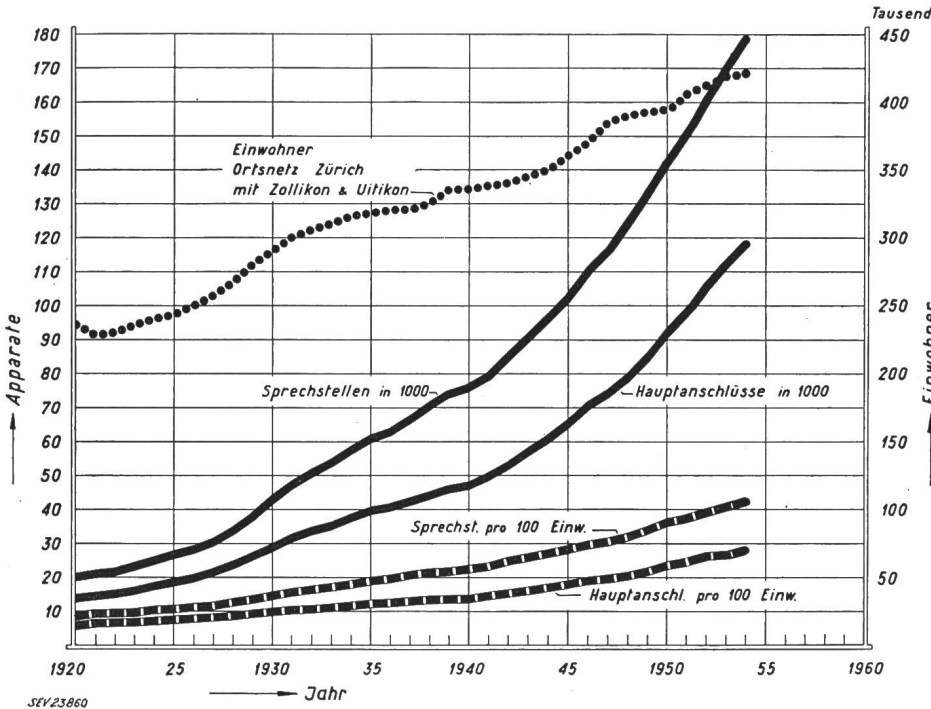
Fig. 1 Entwicklung der Telephon-Hauptanschlüsse und der Sprechstellen im Ortsnetz der Stadt Zürich in den Jahren 1920...1954, verglichen mit der entsprechenden Zunahme der Einwohnerzahl
