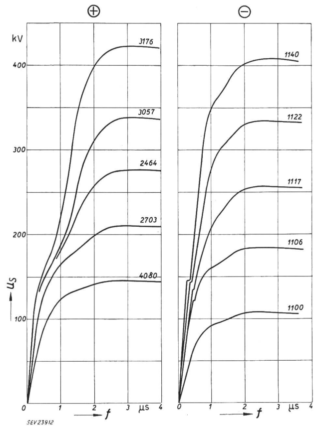
Fig. 9 Front de l'onde de tension ayant parcouru 1 km de ligne Les deux conducteurs câblés de la ligne sont couplés en parallèle. Retour du courant par le sol. t Temps; u_s Onde de tension
