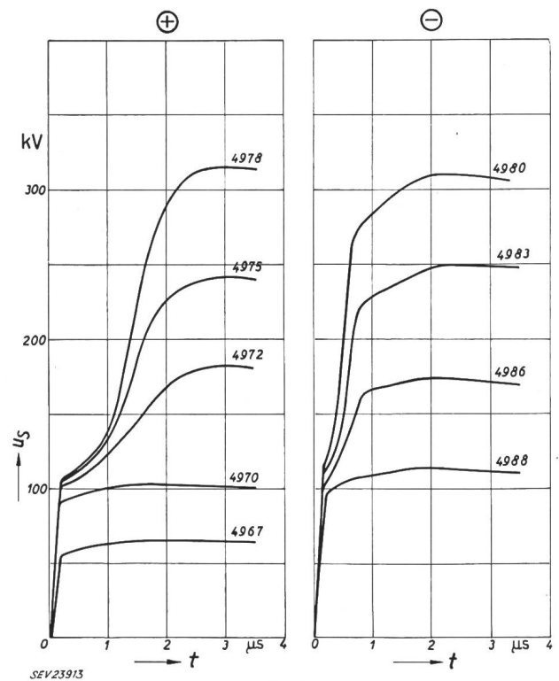
Fig. 10 Front de l'onde de tension ayant parcouru 1 km de ligne L'un des deux conducteurs câblés de la ligne est couplé en parallèle avec le sol servant de conducteur de retour (tension à partir de laquelle se produit un effet de couronne, env. 100 kV) t Temps; u_s Onde de tension
