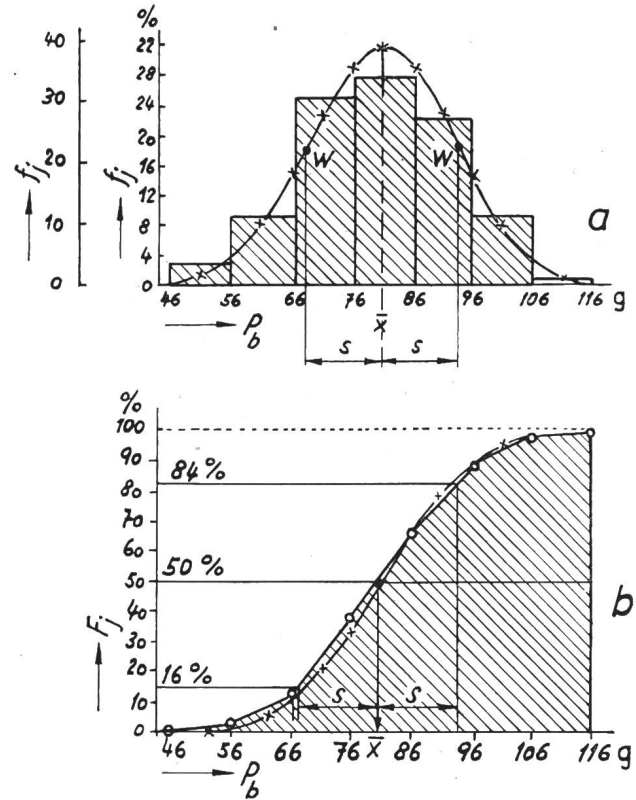
SEV 23 926 Fig. 1 Diagramme des fréquences a et diagramme des fréquences cumulées b pour la détermination de la résistance d'un fil textile f_j fréquence; F_j fréquence cumulée; P_b charge de rupture; W points d'inflexion — allure théorique — — — allure pratique \bar{x} = 80,6 g s = 12,5 g
