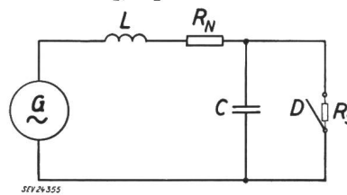
Fig. 13 Schéma équivalent du circuit parcouru par le courant lors des essais
