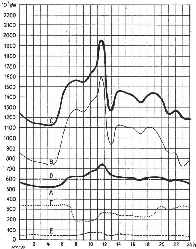
Diagramme de charge journalier du mercredi (Entreprises livrant de l'énergie à des tiers) Mercredi 14 mars 1956
