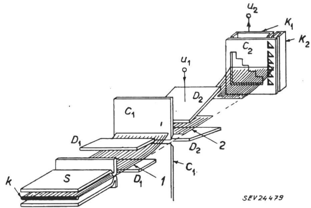
Fig. 3 Prinzipieller Aufbau u_1 Eingangssignal; u_2 quantisiertes Ausgangssignal; 1 Flachstrahl; 2 gestauter Strahl; S strahlerzeugendes System; k Kathode; D_1, D_2 Ablenkplatten; C_2 Blende für die Quantisierung und Signaltrennung; K_1 quantisierter Kollektor (Auffangelektrode); K_2 Restkollektor
