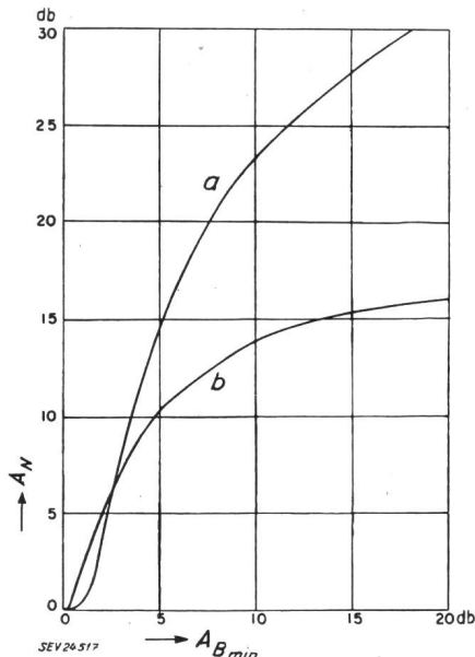
Minimale Betriebsdämpfung in Funktion der Nachbarkanal-dämpfung für a einfache und b doppelt abstimmbare Kreise A_N Dämpfung des Nachbarkanal ( \Delta f \pm 10 kHz); A_{Bmin} minimale Betriebsdämpfung (bei einer ZF von 455 kHz); Leerlauf-Gütefaktor Q_0 = 160
