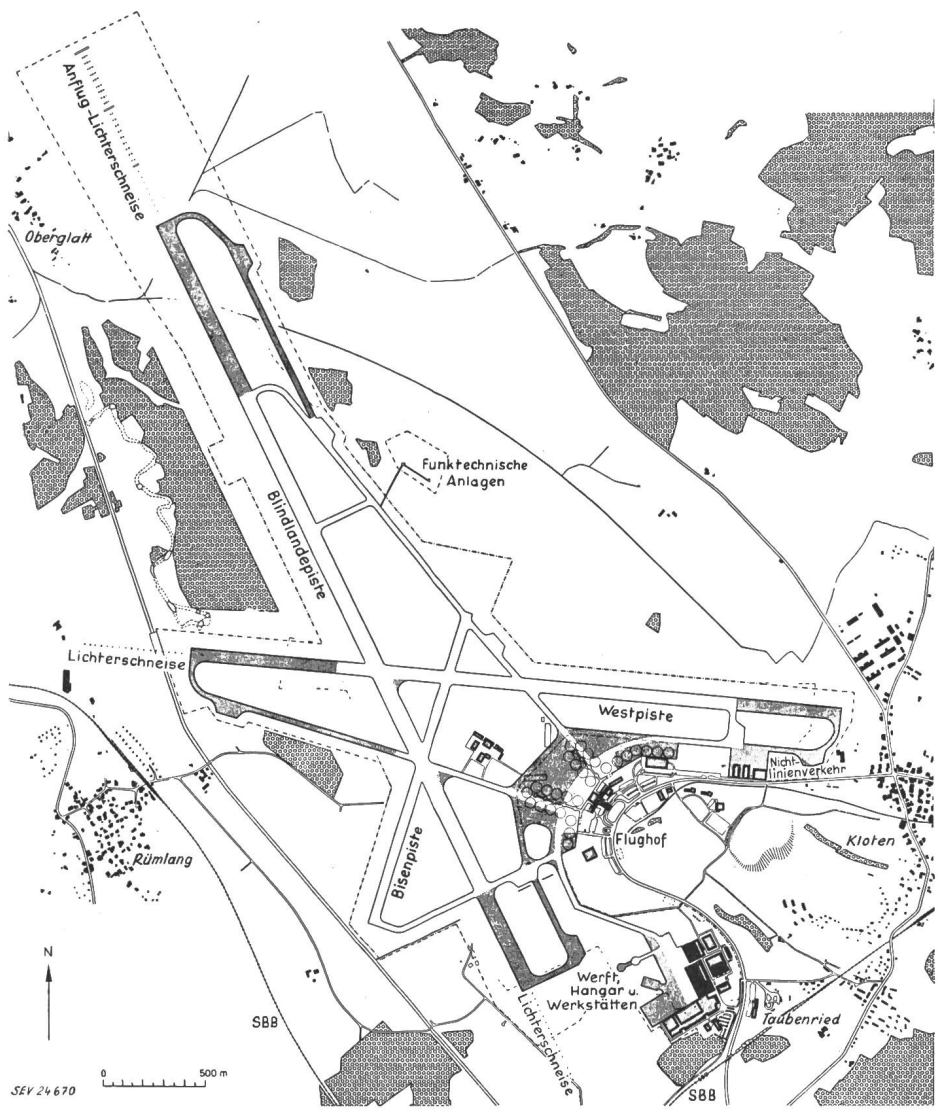
Fig. 1 Interkontinentaler Flughafen Zürich-Kloten Lageplan; 1. und 2. Bauetappe 1. Bauetappe: bestehende Anlagen □ Pisten und Rollwege, Flugsteig ■ Gebäude 2. Bauetappe: projektierte Anlagen □ Pisten und Rollwege, Flugsteig □ Gebäude
