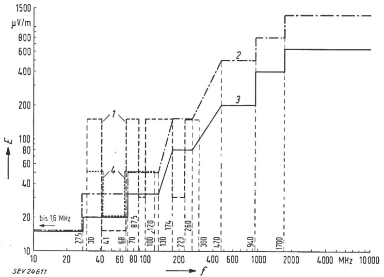
Fig. 2 Grenzwerte der Störfeldstärke E für Ton- und Fernsehempfänger
