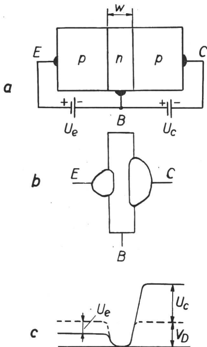
Fig. 12 p-n-Transistor
