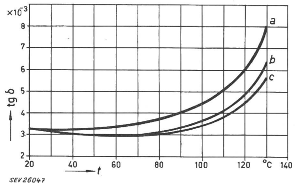
Fig. 5 Temperaturabhängigkeit des Verlustfaktors bei verschiedenen Messfeldstärken eines einwandfreien Kondensators Feldstärken: a 2 V/μ; b 8 V/μ; c 14 V/μ
