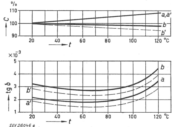
Fig. 4 Verlustfaktor \text{tg } \delta und Kapazität C von Papieren verschiedener Satinage in Funktion der Temperatur a vakuumgetrocknete, unimprägnierte Wickel, Satinage A b mit Pyralène 1476 imprägnierte Wickel, Satinage A a' vakuumgetrocknete, unimprägnierte Wickel, Satinage C b' mit Pyralène 1476 imprägnierte Wickel, Satinage C
