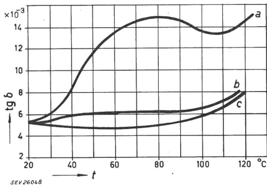
Fig. 6 Wie Fig. 5, aber mit verunreinigten Imprägniermitteln
