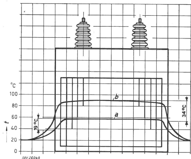
Fig. 7 Temperaturverteilung in einem Kondensator nach Fig. 11 bei zwei verschiedenen Spannungen a bei einer Spannung von 3000 V; b bei einer Spannung von 4000 V
