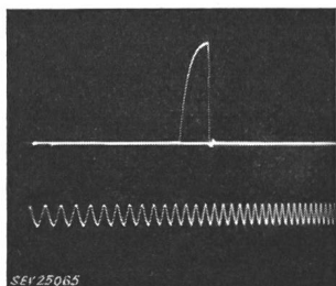
Fig. 6 Nach 1 \mu s abgeschnittene Stossweite Eichfrequenz 2 MHz
