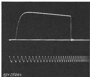
Fig. 5 Nach 9 \mu s abgeschnittene Stossweite Eichfrequenz 2 MHz
