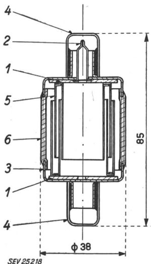
Fig. 18 Schnitt durch einen Vakuumkondensator 1 Stahlplatte; 2 Saugstutzen; 4 Kappe; 5 innere Elektrode; 6 Glaskörper
