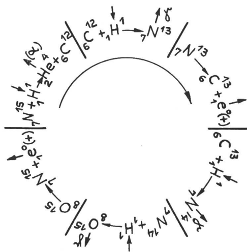
SEV 25080 Fig. 6 Chaîne cyclique des réactions du soleil
