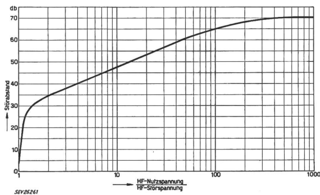
Fig. 9 Unterdrückung eines Störsenders durch den stärkeren Nutzsender
