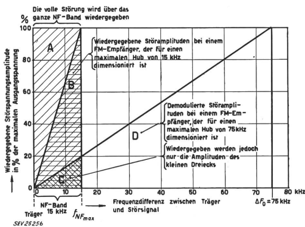
Fig. 4 Das «Stördreieck»
