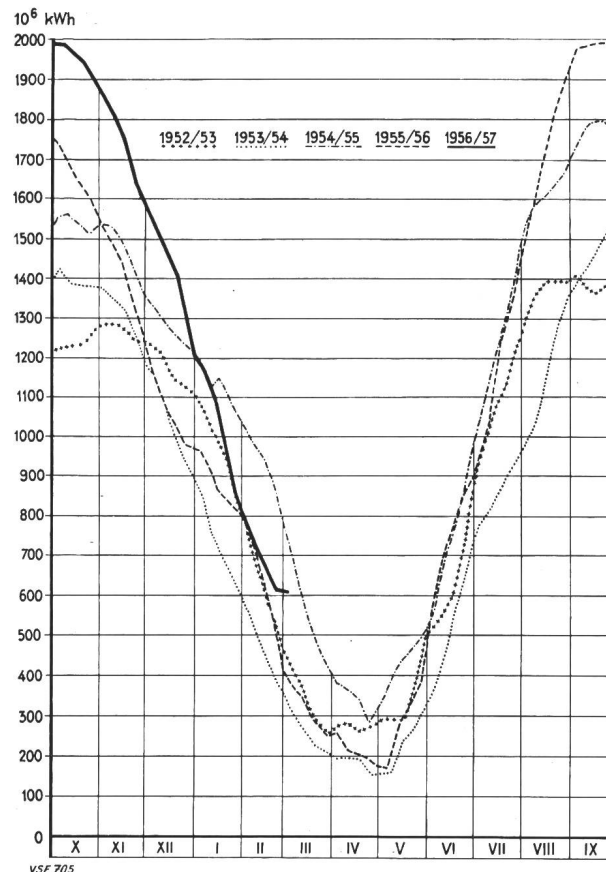
Fig. 5 Réserve d'énergie emmagasinée dans l'ensemble des bassins d'accumulation
