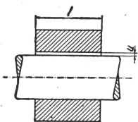
Fig. 3 Longueur du joint l et jeu diamétral u dans le cas d'arbres tournants
