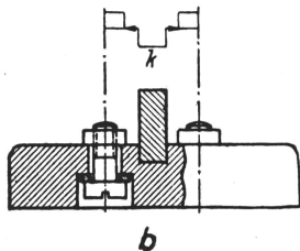
Fig. 8 Subdivision des lignes de fuite par nervure (a) ou traverse (b)
