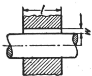
Fig. 4 Longueur du joint l et interstice w entre axe et alésage (parties se déplaçant occasionnellement l'une par rapport à l'autre)
