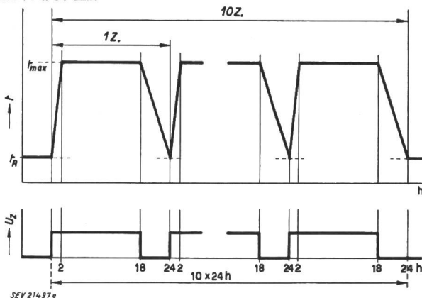
Fig. 8 Surcharge cyclique de condensateurs t Température. t_R Température ambiante. t_{max} Température superficielle maximum. Z Cycle. U_z Tension d'essai.
