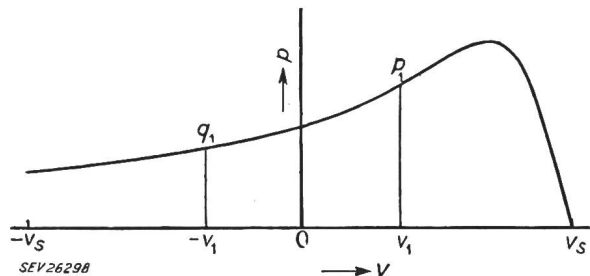
Fig. 2 Kraft-Geschwindigkeitskurve des geradlinigen Motors p Kraft; v Geschwindigkeit Weitere Bezeichnungen siehe im Text
