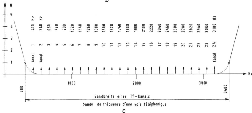
Spectre de fréquences d'une voie de télégraphie harmonique et schéma de principe de l'émetteur et du récepteur d'une extrémité de voie
