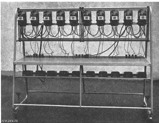
Fig. 2 Eichgestell im Betrieb
