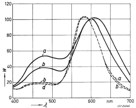
Fig. 12 Wie Fig. 11, aber für die Farbtongruppe «Warmweiss» a Osram «Warmweiss»; b Westinghouse «soft white» Weitere Bezeichnungen siehe Fig. 11
