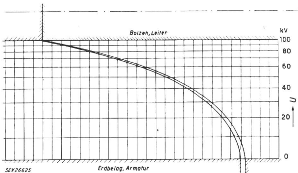
Fig. 3 Feldbild einer Fugenkupplung U Spannung
