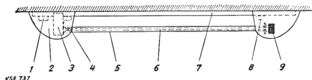
Fig. 4 Avertisseur différentiel et limitatif combiné 1 boîte de jonction; 2 capsule de contact; 3 contact; 4 dispositif de déclenchement à maximum de température; 5 tube métallique extérieur; 6 tube métallique intérieur; 7 socle; 8 suspension à ressort; 9 vis de réglage
