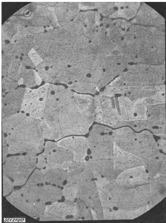
Fig. 1 Wasserstoffkrankes Kupfer, das sich beim Löten mit Silberlot vollgesogen hat Vergrößerung 200fach
