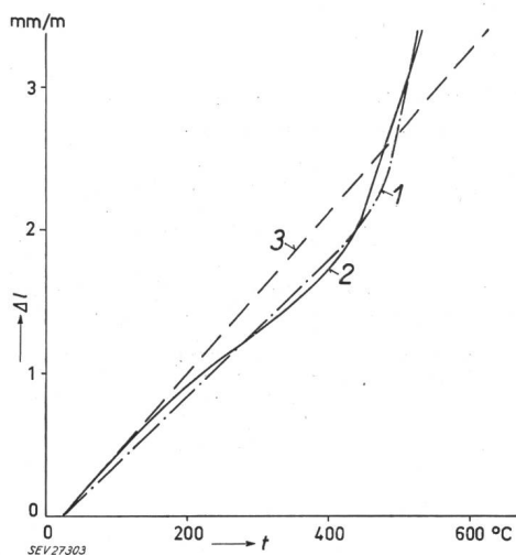
Fig. 3 Ausdehnung von Kovarglas (1), Kovar (2) und Molybdän (3) \Delta l Ausdehnung; t Temperatur
