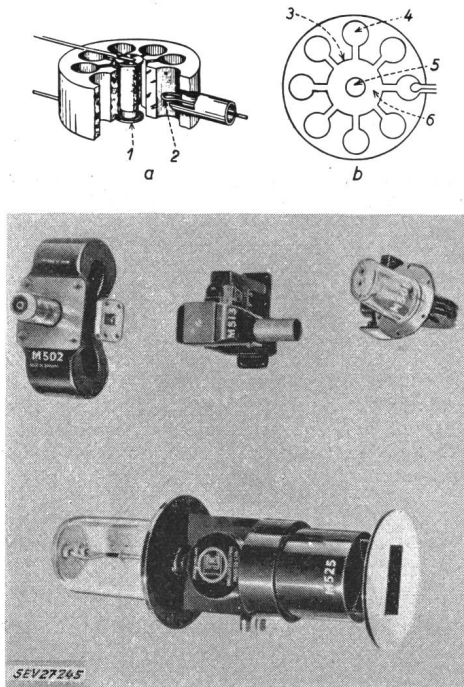
Fig. 11 Magnetron
