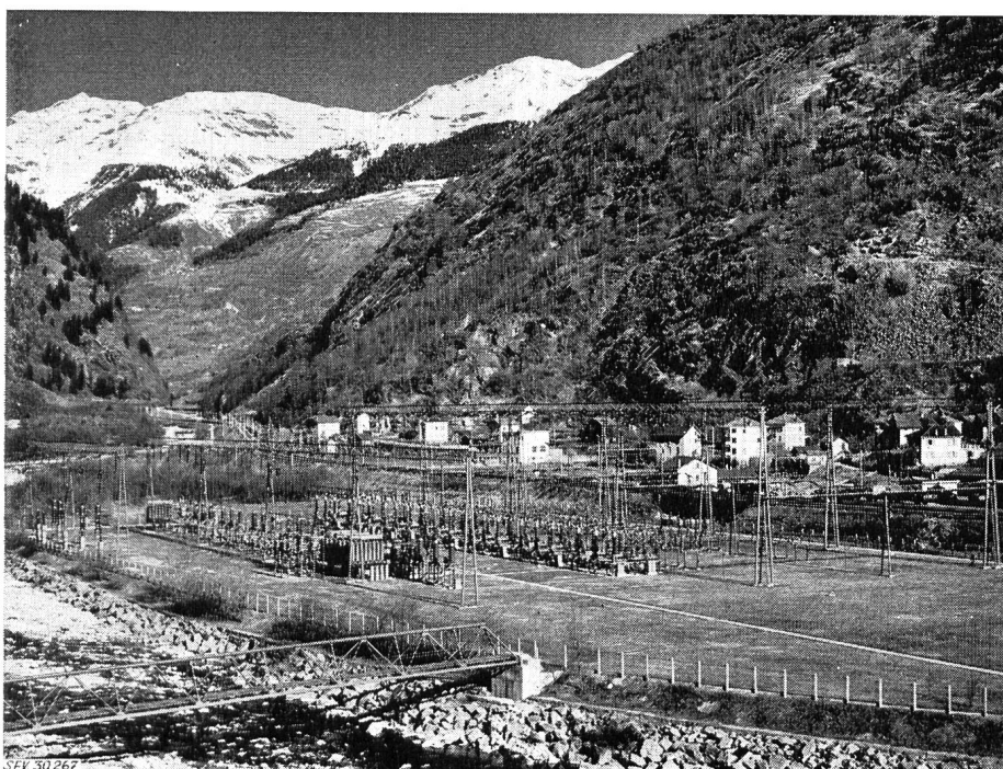
Ansicht der Station Lavorgo zwischen dem Fluss Tessin und der Eisenbahn
