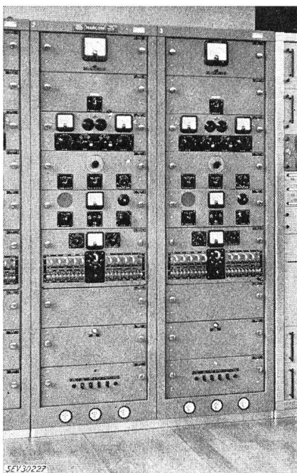
Fig. 7 Générateurs de BLU Centre émetteur de Münchenbuchsee
