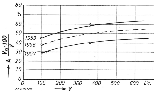
Fig. 8 Zunahme der Raumaussnutzung bei Haushalt- und Gewerbekühlschränken durch bessere Konstruktionen und verbesserte Kälteschutzstoffe
