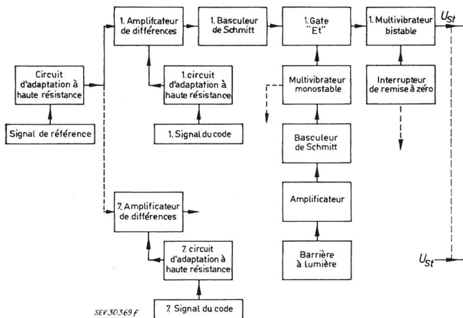
Fig. 9 Schéma de principe de l'appareil de lecture U_{st} signal de commande
