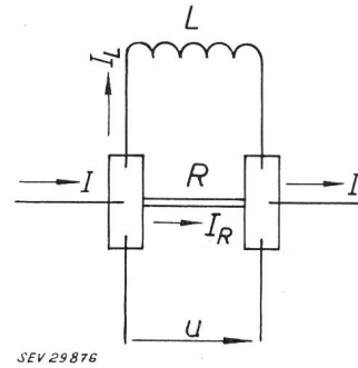
Fig. 1 Schematische Darstellung eines Persistor-Speicherelementes
