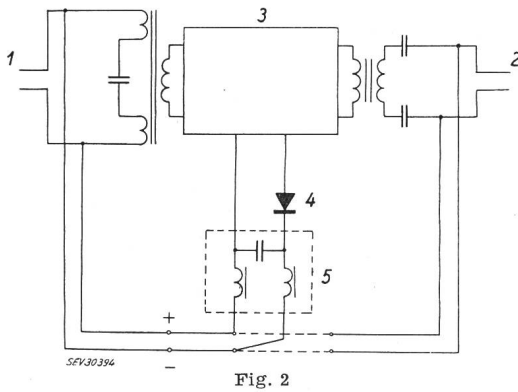
Fig. 2 Gleichstromspeisung des Verstärkers
