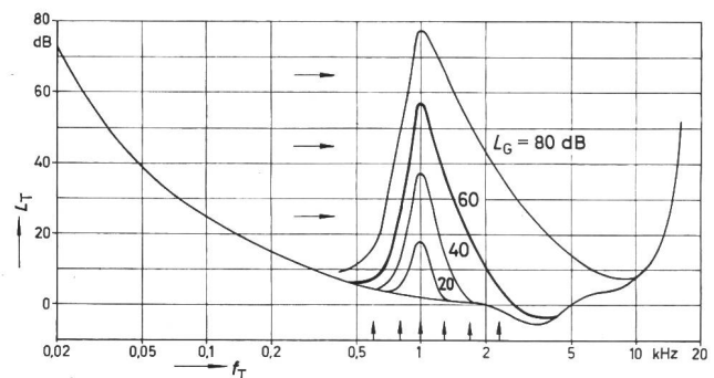
Fig. 6 Mithörschwelle L_T von Sinustönen verdeckt durch frequenzgruppenbreites Schmalbandrauschen mit dem Pegel L_G und der Mittenfrequenz 1 kHz als Funktion der Frequenz f_T des Testtones
