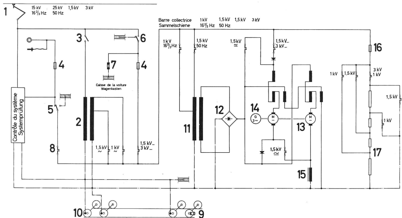
Fig. 4 Circuits principaux
