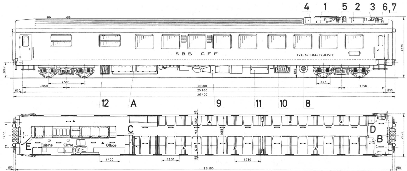
Fig. 1 Dessin type
