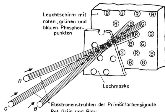
Fig. 5 Arbeitsweise der Lochmaskenröhre
