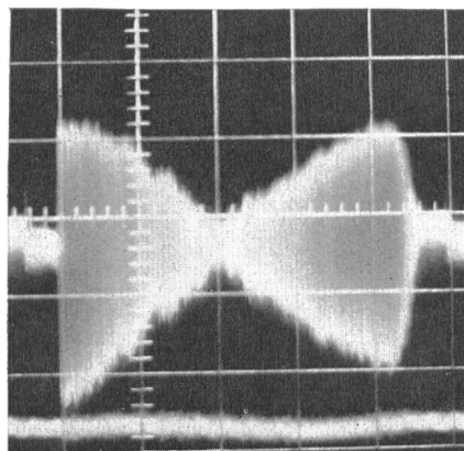
Fig. 21 Empfang des Fernsenders Niederhorn beim Bahnhof Spiez Videofrequentes Spektrum als Funktion der Masthöhe der Antenne (10-Element-Yagi-Typ), mit starkem ortsabhängigen Selektivschwund; Frequenzbereich: 0,5...5 MHz (Wobbelsignal). Die Masthöhen lagen im Bereich 7...10 m.
