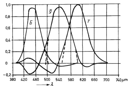
Fig. 6 NTSC-Farbmischkurven für die Aufnahme-seite \bar{b} blau; \bar{g} gelb; \bar{r} rot; \lambda Wellenlänge
