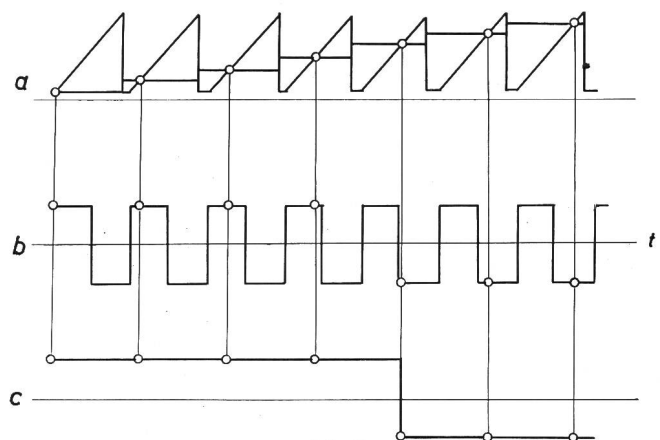
Fig. 2 Fonctionnement de l'appareil d'essai a dent de scie, escalier; b signal d'entrée; c signal de sortie; t temps
