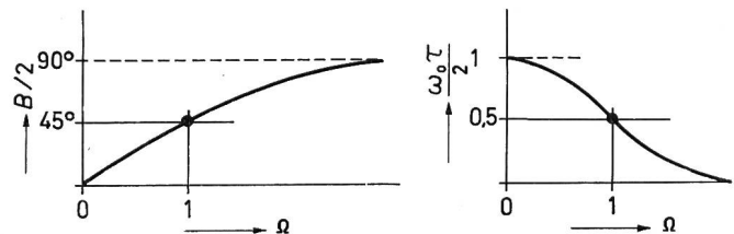
Fig. 5 Phasen- und Laufzeitfunktion beim Grundglied 1. Ordnung \Omega = \omega/\omega_0 normierte Frequenz
