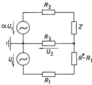
Fig. 17 Allpass-Netzwerk, das durch zwei gegenphasige Quellen angesteuert wird
