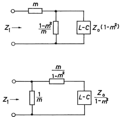
Fig. 15 Realisierungsmöglichkeiten für die RLC-Impedanz Z_1 , ausgehend von der verlustlosen LC-Impedanz Z_0 und dem Parameter m Erklärungen siehe im Text
