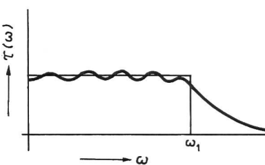
Fig. 3 Approximation einer konstanten Verzögerung Die praktische Laufzeitfläche wird etwas grösser als die vorgegebene Rechteckfläche \tau(\omega) Laufzeit; \omega_1 Grenzfrequenz
