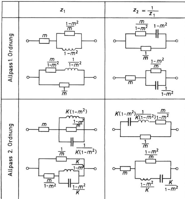
Fig. 16 Allpassimpedanz z_1 und ihre Dualimpedanz z_2
