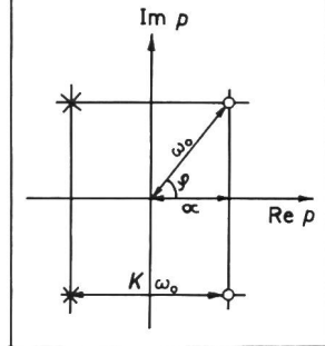
Fig. 15 Realisierungsmöglichkeiten für die RLC-Impedanz Z_1 , ausgehend von der verlustlosen LC-Impedanz Z_0 und dem Parameter m Erklärungen siehe im Text
