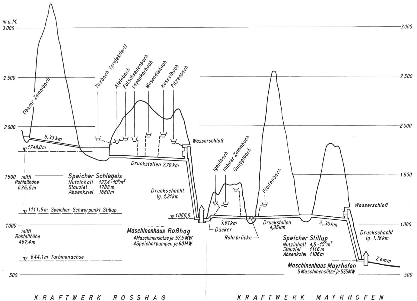
Fig. 1 Höhenschnitt der Zemmkraftwerke
